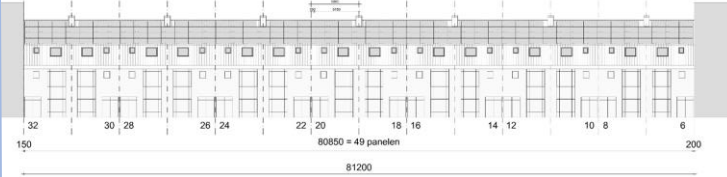
NIEUWE voorgevel Kraaipanstraat 6 t/m 32 met zwarte zonnepanelen op het bovenvlak
