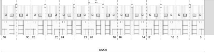
BESTAANDE voorgevel Kraaipanstraat 6 t/m 32
