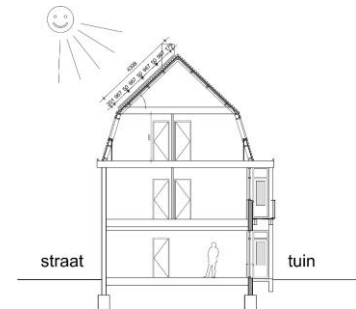
Doorsnede met zonnepanelen
